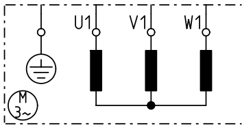
Sternschaltung/star wiring
