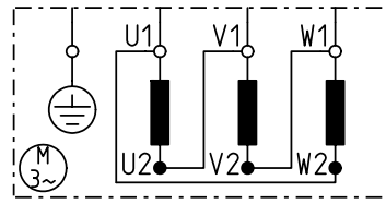
oder/ Dreieckschaltung/delta wiring
