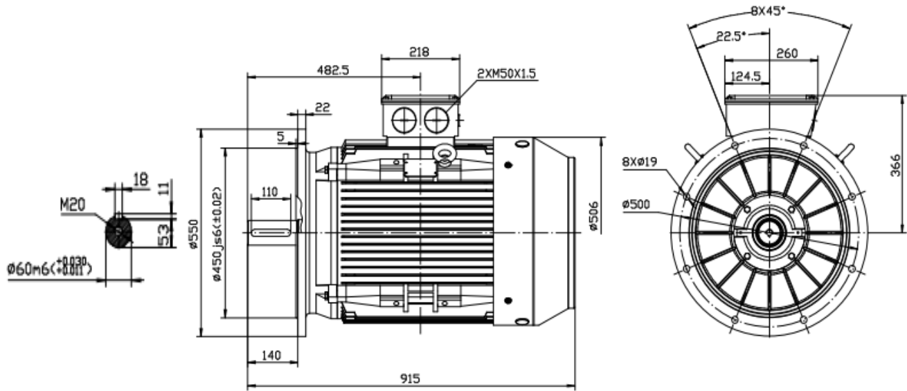
Typ / type IE3 SEV- 250M-2
