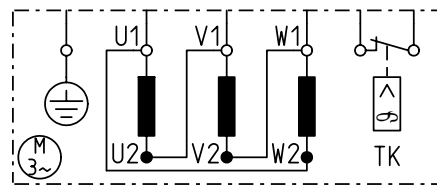
Dreieckschaltung/delta wiring
