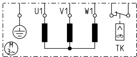
Sternschaltung/star wiring
